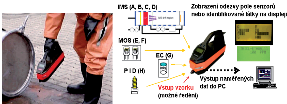
Obr. 7.23 Analyzátor nebezpečných plynů a par a bojových otravných látek GDA 2
