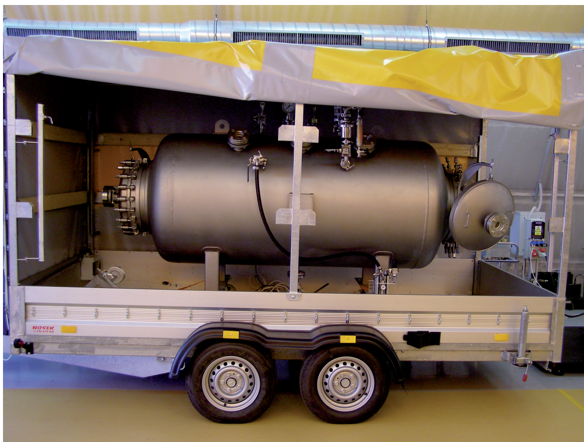
Ilustrační foto: Bezpečnostní transportní přetlaková plynotěsná komora s manipulátorem
