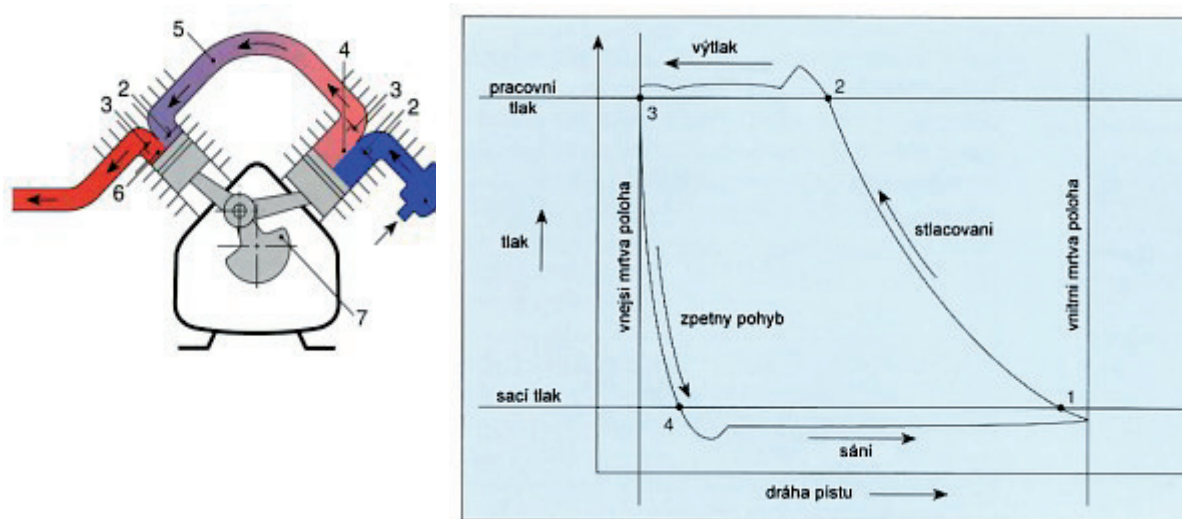
Obr. 5.1 Popis funkce dvoustupňového kompresoru
