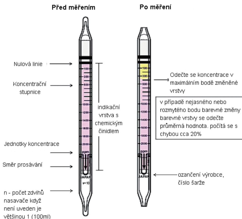
Obr. 7.11 Princip délkové detekční trubičky
