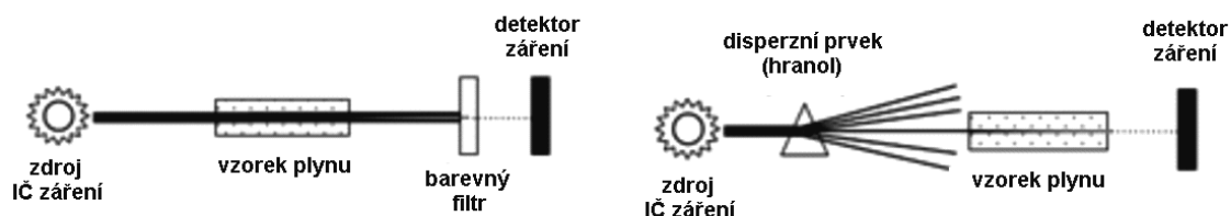
Obr. 7.10 Porovnání principu NDIR (nedisperzní, vlevo) a DIR (disperzní, vpravo)
