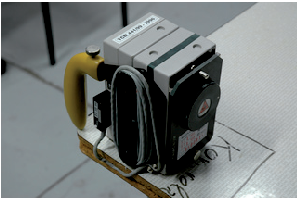
Umístění radiometru DC-3E-98 při provádění kontroly na etalon
