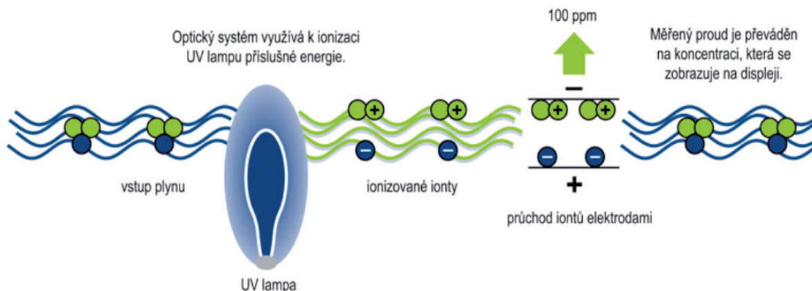
Obr. 7.8 Princip fotoionizačního detektoru
