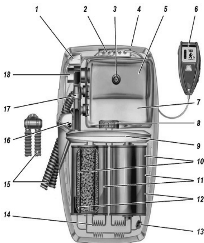
Obr. 3.23 Schéma kyslíkového dýchacího přístroje Air Elite: 1 – akumulátor, 2 – elektrický rozvaděč, 3 – přetlakový ventil (zadní strana dýchacího vaku), 4 – zdířka pro nabíjení, 5 – výdechový vak, 6 – IC-Air, 7 – nádechový vak, 8 – filtr na zachycování částic, 9 – rozdělovač vzdušiny, 10 – chladič plášť, 11 – kanystr s chemikálií (2x), 12 – rychlostartér (2x), 13 – přípojka kabelu startéru, 14 – vedení chladičem, 15 – sada dýchacích hadic, 16 – senzorová jednotka, 17 – přepážka se směrovými ventily, 18 – ventilátor – přípojka masky na startovací automat (na levém ramenním popruhu)
