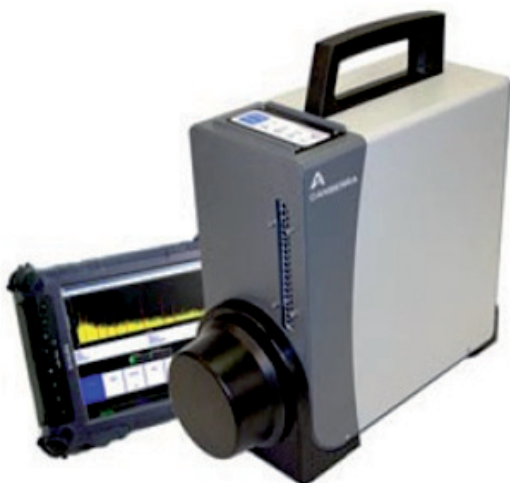
Obr. 9.9 Mobilní polovodičový gama spektrometr Falcon 5000 N a měřič kontaminace alfa, beta, gama Contamat FHT 111H
