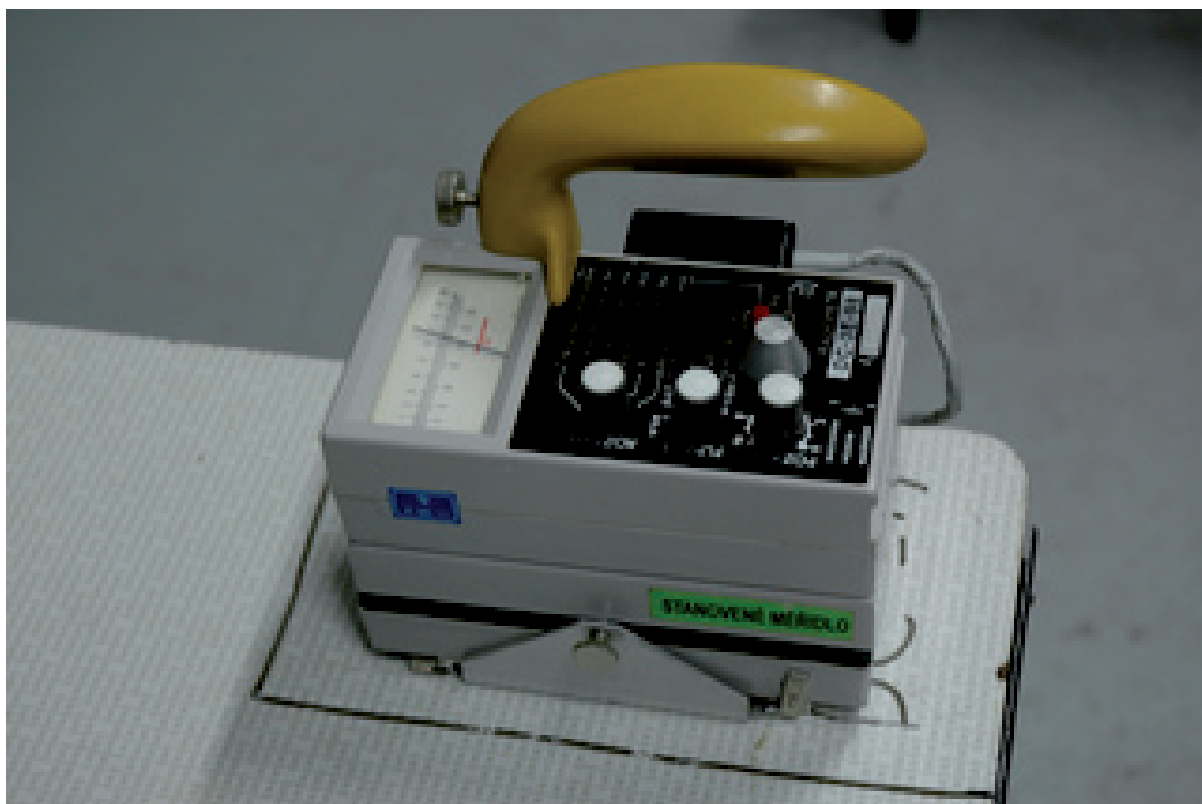
Umístění radiometru DC-3E-98 při provádění kontroly pozadí na pracovním stole
