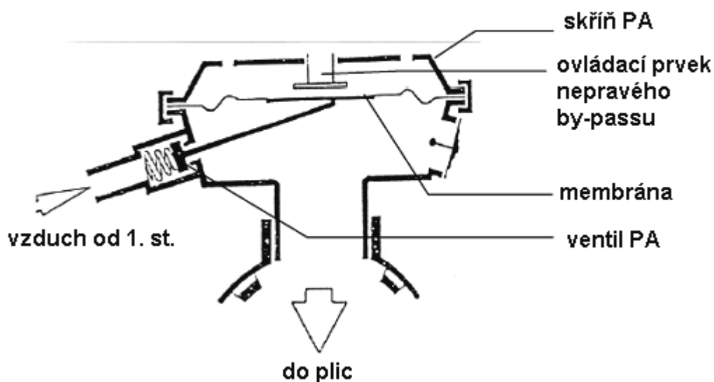
Obr. 3.13 Řez přetlakovou plicní automatikou s vyvracecí kuželkou
