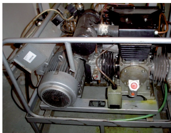
Obr. 5.5 Vysokotlaký kompresor Trident
