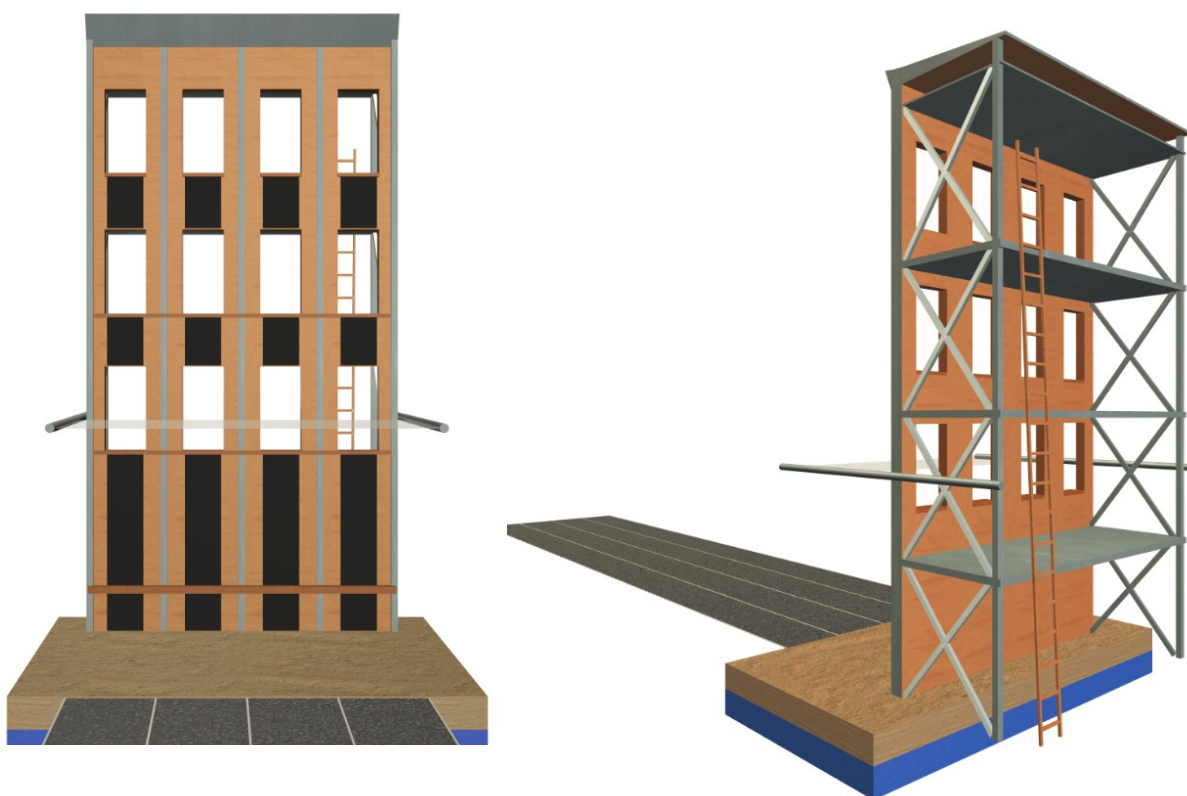
Schéma uspořádání bezpečnostní sítě
