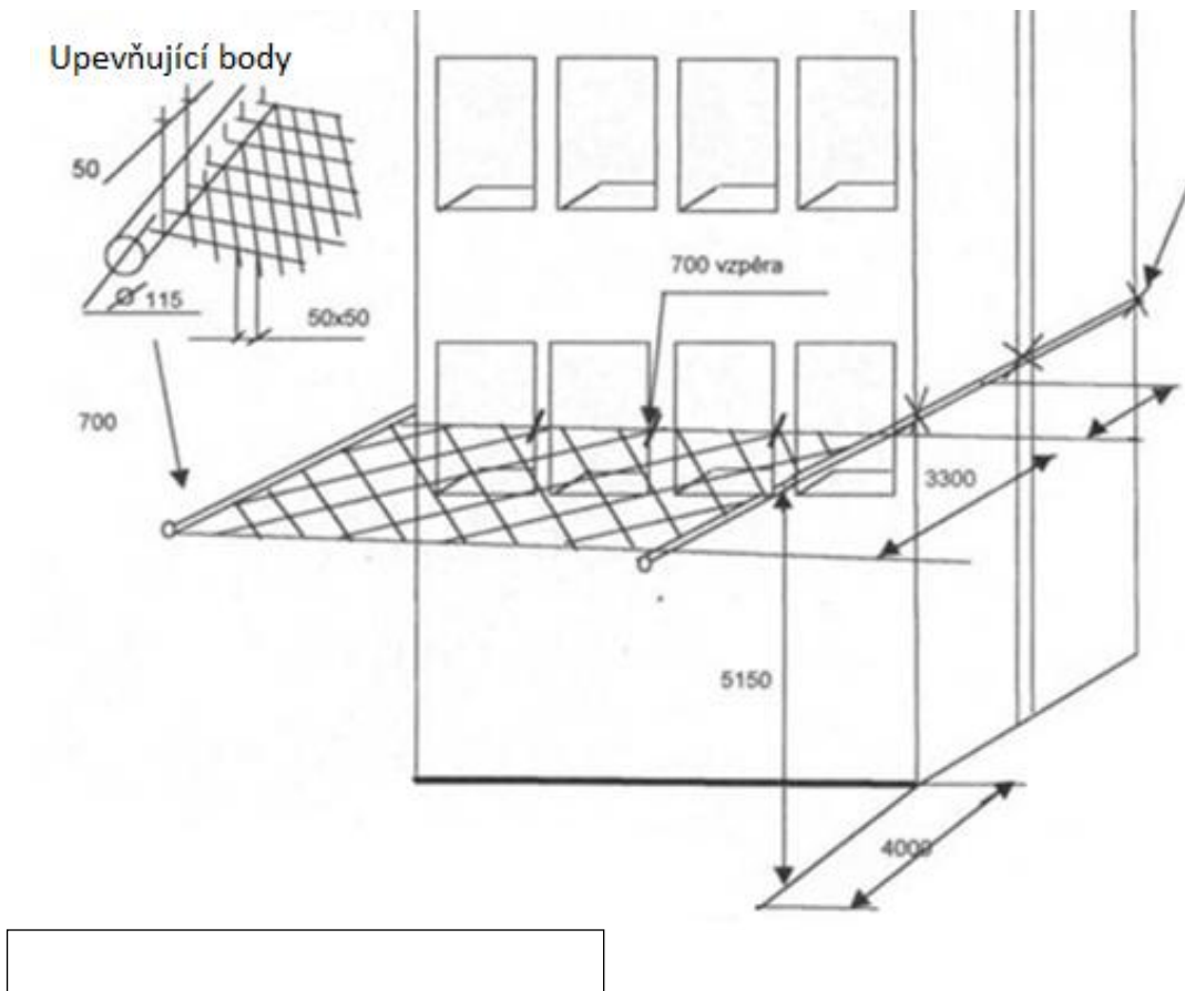
Schéma uspořádání bezpečnostní sítě
