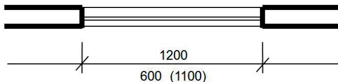
Obr. 14 Kótování oken
