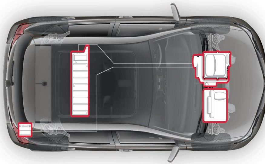
Obrázek 8 – Umístění baterie u hybridu [15]
