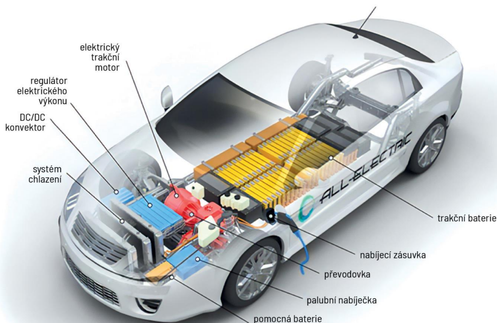
Obrázek 6 – Schéma elektrovozidla [13]
