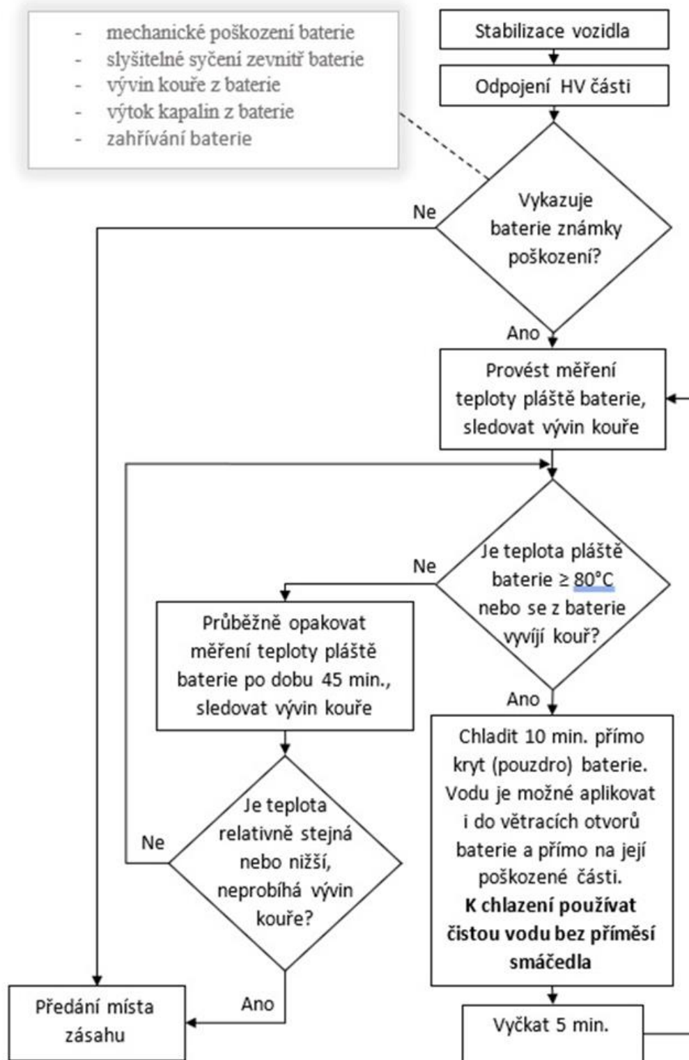
Obrázek 24 – Algoritmus chlazení trakční baterie vodním proudem
