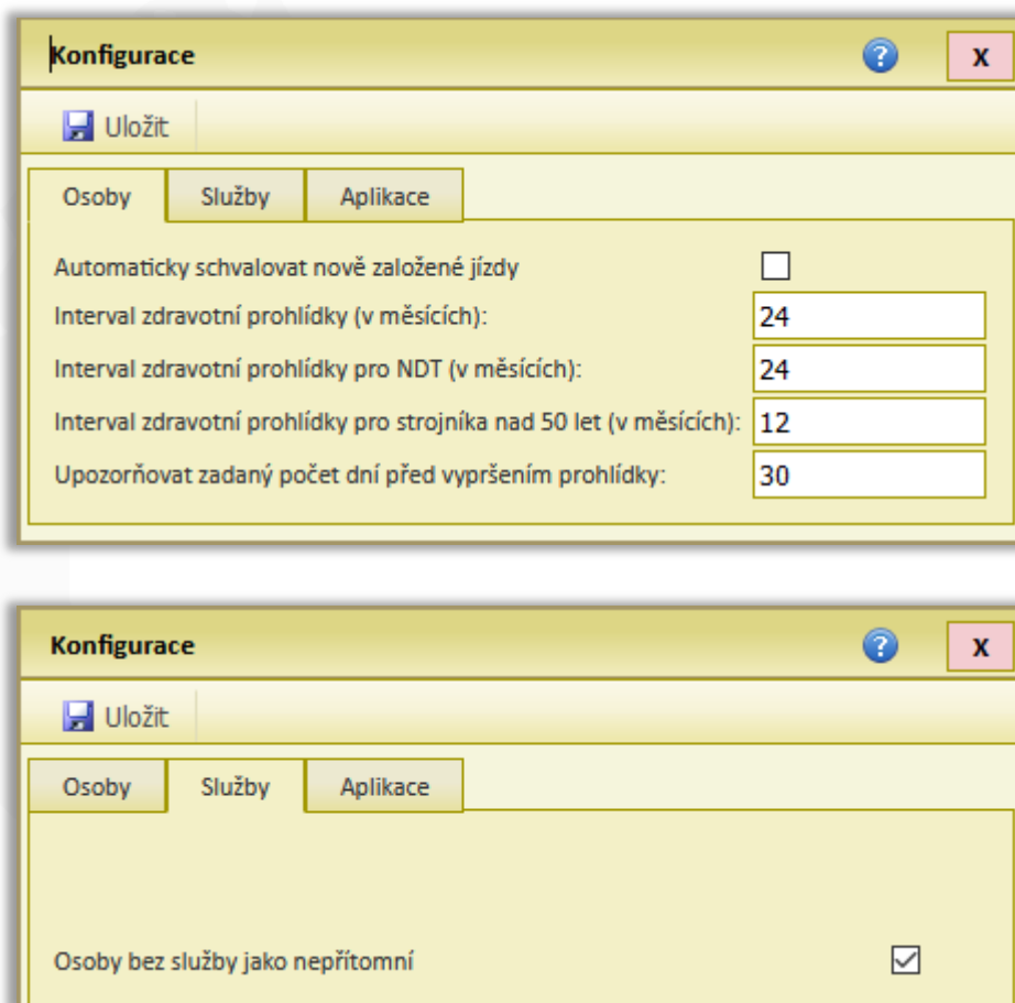
Obrázek 102: konfigurace aplikace
